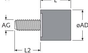
Gerätefüße / Schwingungsdämpfer Mounting feet / vibration dampeners
