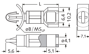
Kunststoff-Distanzhalter, einrastend, Fixierung durch Spreizniete Snap-lock + snap-rivet plastic PCB spacers
